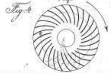
Ansicht der Mahlfläche des Läufers der Steinmühle im Dampfdruckwerk u. Binnschiffahrt
