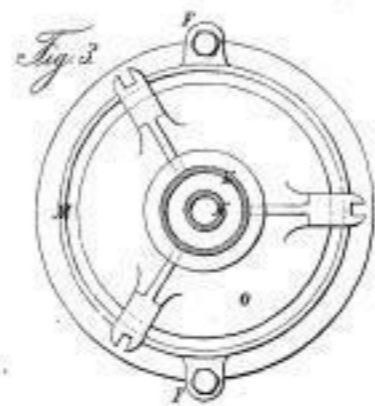
Ansicht der Mahlfläche des Läufers der Steinmühle im Dampfdruckwerk u. Binnschiffahrt
