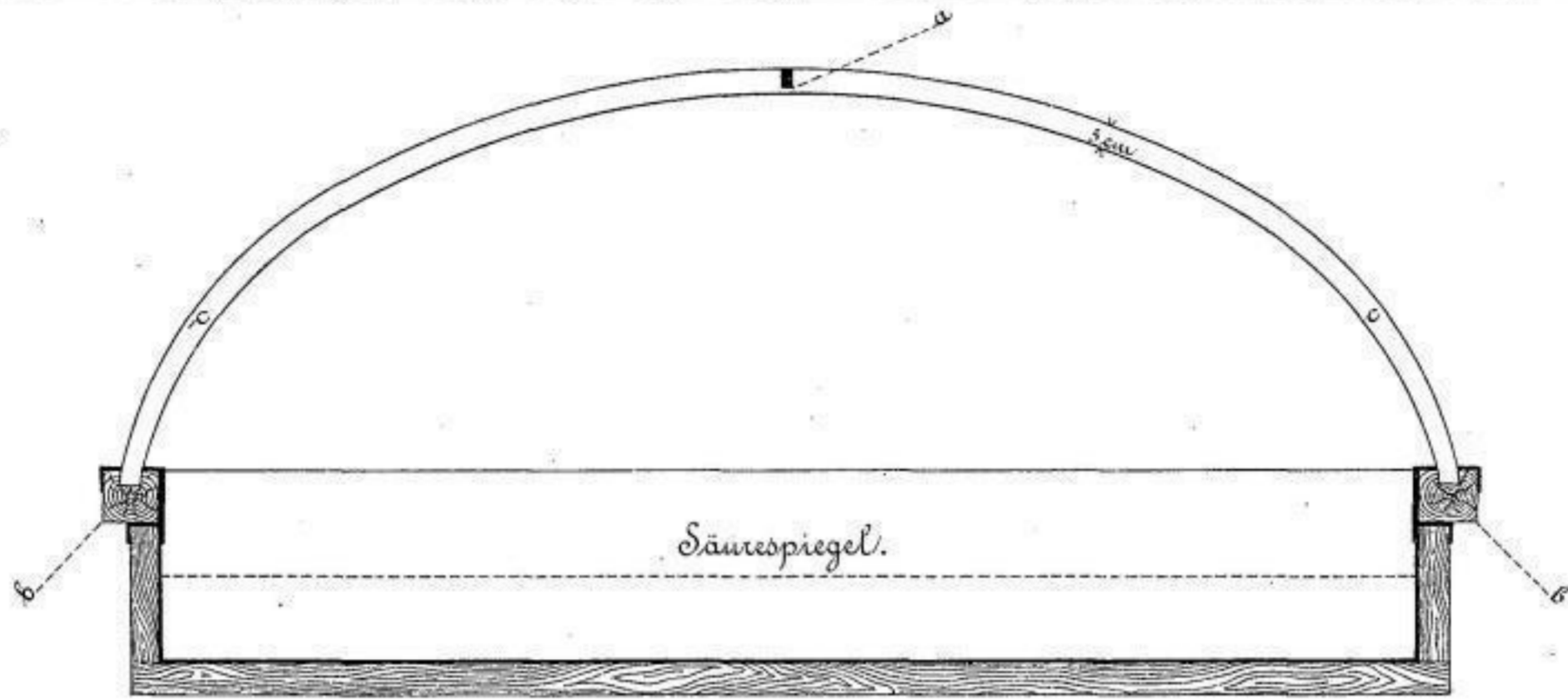
Fig. 3: Schnitt nach C-D. \frac{1}{200} der nat. Grösse.
